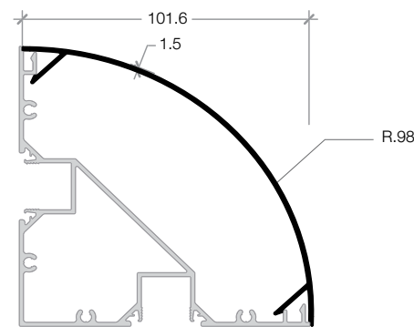
T-02C CONNER DOME SHAPE เสาโค้ง 100 มม.
