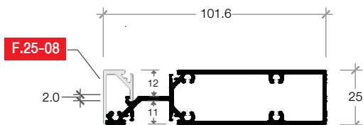
T-25.17 FRONT LINE TRANSOM FRAME ซอยลูกฟักร่องข้าง 25 มม.
