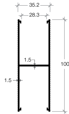
P-03 T5-ALU BATTEN รางไฟ 100 มม. x 35 มม.
