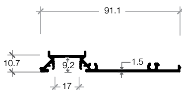
T-25.14 FRONT LINE SNAPPING MULLION ตบกล่องร่องข้าง 25 มม. ใช้คู่กับ T-25.13
