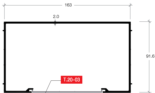
P-01 POWERPOLE FOR ACCESS CONTROL เสาสำหรับงานระบบไฟ 163 มม. x 91.6 มม.
