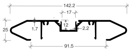
T-25.03P MULLION 25 mm. กล่องร่องมีปีกข้าง 25 มม.
