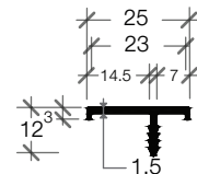
D-25 ALU-DEC FOR WOOD DOOR ปิดสันบานประตู 25 มม.
