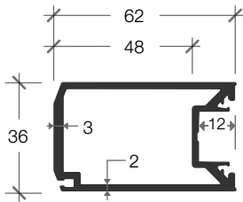
D-60 VERTICAL DOOR 60 MM. เสาประตู 60 มม.
