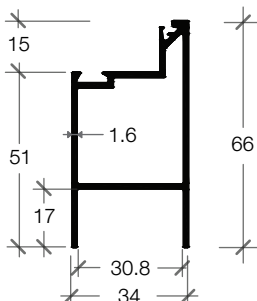
D-63A TOP SWING DOOR วางประตู บานเปิด
