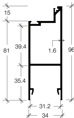
D-64 BOTTOM DOOR วางล่างประตู
