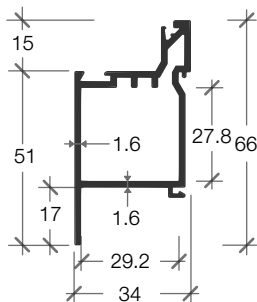
D-63 TOP SLIDING DOOR วางประตูบานเลื่อน
