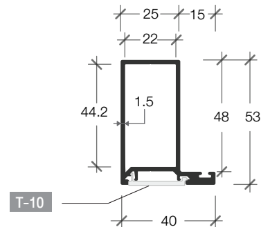
D-67 ALUMINIUM BOX เสารับบานประตู 35 - 45 มม.
