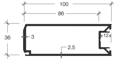
D-100 VERTICAL DOOR 100 MM. เสาประตู 100 มม.
