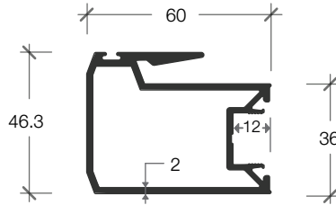
D-60S JOINT DOOR เสาเกี่ยว 60 มม.
