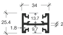
D-69 HORIZONTAL MULLION ซอยลูกฟักประตู 25 มม.
