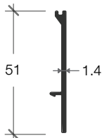
D-61 SNAPPING TOP DOOR ฝาปิดวางประตู 35 มม. ใช้คู่กับ D-63
