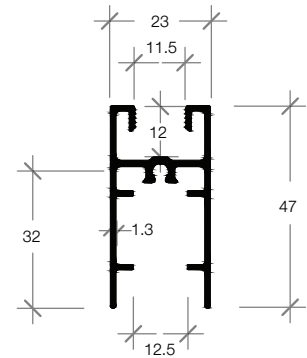
E-07E TOP & BOTTOM WINDOW FRAME วงงหน้าต่าง
