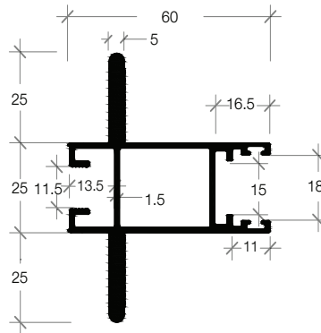
E-04GP DOOR FRAME WITH HANDLE เสาทุกุญแจใส่เกียร์มีมือจับ
