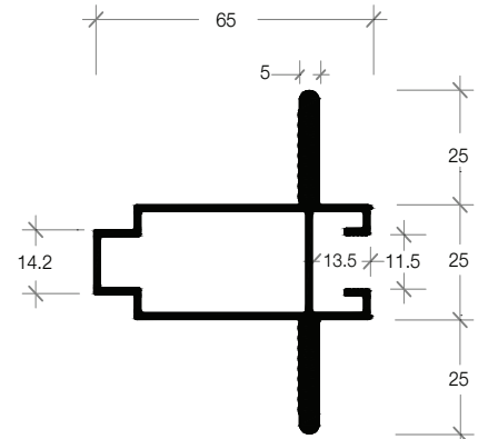
E-04HH DOOR FRAME WITH 2 HANDLE เสาเหลี่ยมมีมือจับ 2 ทาง
