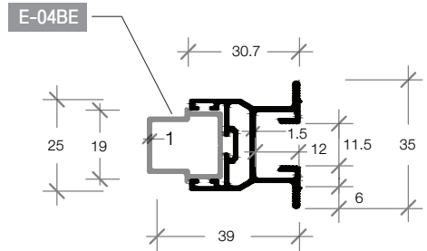
E-04E WINDOW FRAME KEY เสากุญแจมือจับหน้าต่าง
