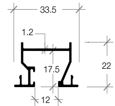
E-01F FIX GLASS TOP RAIL ตรึงกระจกบน
