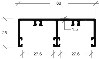
E-01E TOP RAIL 2 TRACK รางบน 2 ราง
