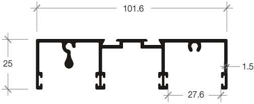
E-01 TOP RAIL 3 TRACK รางบน
