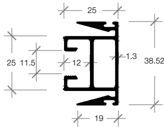
E-06E DOUBLE DRAG WINDOW FRAME เสาทึบหน้าต่าง 2 ทาง
