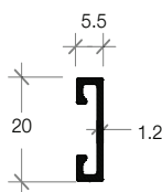
E-09 TRIM FRAME คิ้วชวยหลอก
