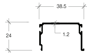
E-03D END OF THE SILLS ฝาปิดบรรณ
