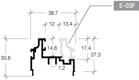
E-03E BOTTOM FIX GLASS ตะรางล่างกล่องเปิด
