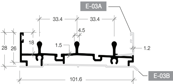
E-03 BOTTOM RAILS 3 TRACK รางล่าง
