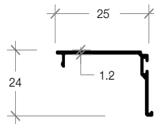
E-03C STRIP OFF SCREEN TRACK ฝาปิดรางมุ้ง
