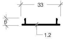
E-01A CLIP TOP RAIL ฝาปิดรางบน
