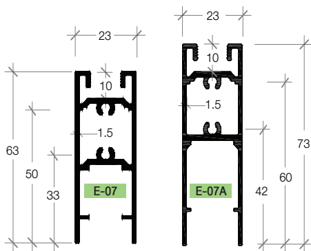
E-07 TOP & BOTTOM DOOR FRAME 1 วางประตูเล็ก 60 . 80 . 160
