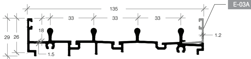
E-03L BOTTOM RAILS 4 TRACK รางล่าง 4 ราง
