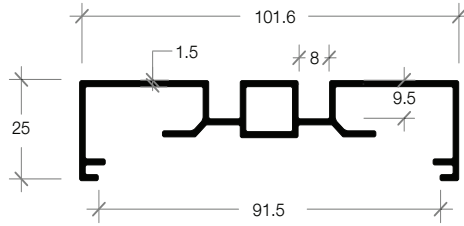
E-02B SIDE RAILS CENTER SLIDING รางข้างร่องกลาง
