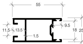
E-04A DOOR FRAME STYLE 1 เสาทุกุญแจ
