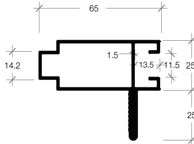
E-04BH DOOR FRAME WITH HANDLE เสาเหลี่ยมมีมือจับ
