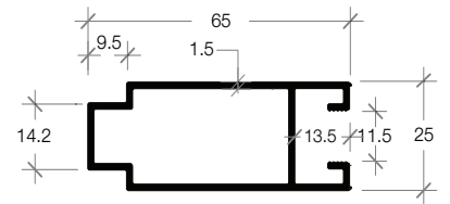
E-04B DOOR FRAME STYLE 2 เสาเหลี่ยม
