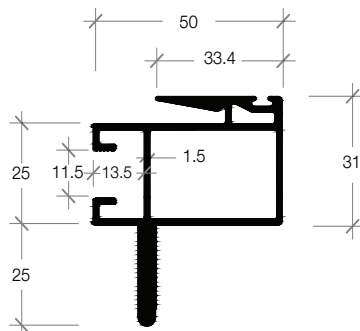
E-05H DOOR FRAME WITH HANDLE เสาเดี่ยวมีมือจับ
