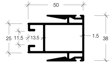
E-06 DOUBLE DRAG DOOR FRAME เสาเดี่ยว 2 ทาง
