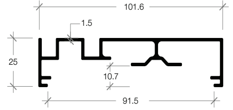
E-02C SIDE RAILS FRONT SLIDING รางข้างร่องรับ
