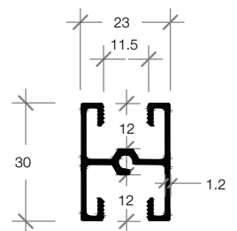
E-10 MID WINDOW FRAME ชวยกลางบานเลื่อน
