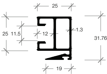
E-05E DRAG WINDOW FRAME เสาทึบหน้าต่าง
