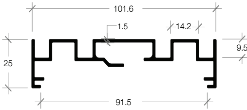
E-02A SIDE RAILS FOR SCREEN รางข้างแบบใส่มุ้ง
