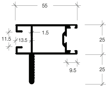
E-04H DOOR FRAME WITH HANDLE เสาทุกขุมมีมือจับ
