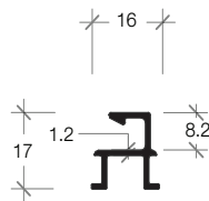
E-08 SCREEN TRIM คิ้วมุ้ง
