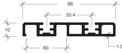
E-03i BOTTOM RAIL 2 TRACK รางล่าง 2 ราง ใช้ภายใน
