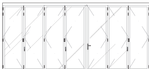
4 : 3 PANEL
