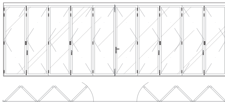
5 : 5 PANEL
